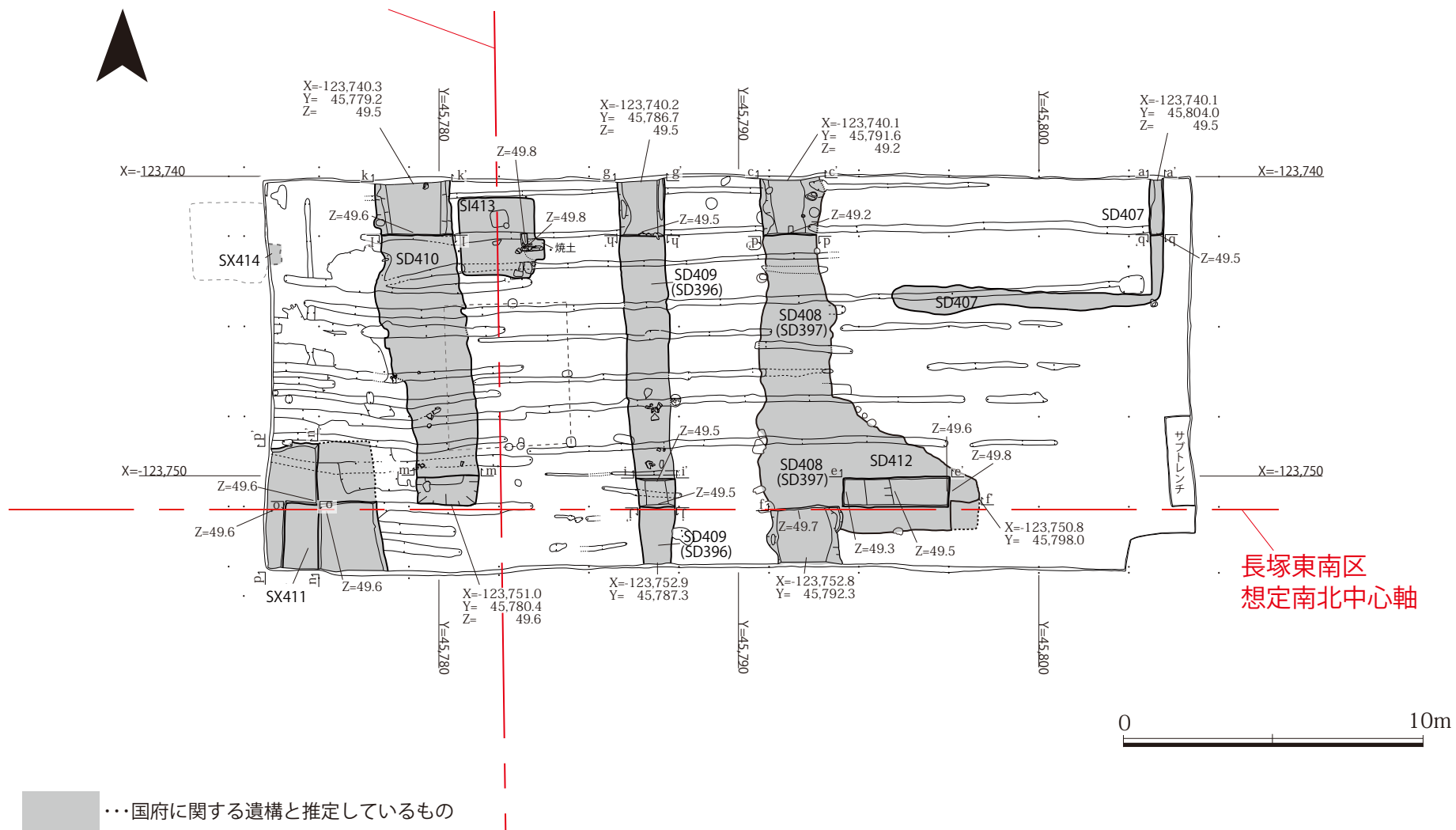
第 45 次調査区平面図 (1 : 200)
