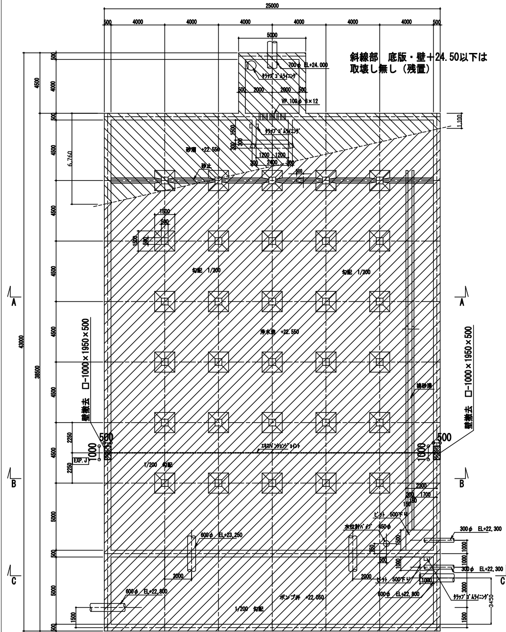
浄水池平面図
