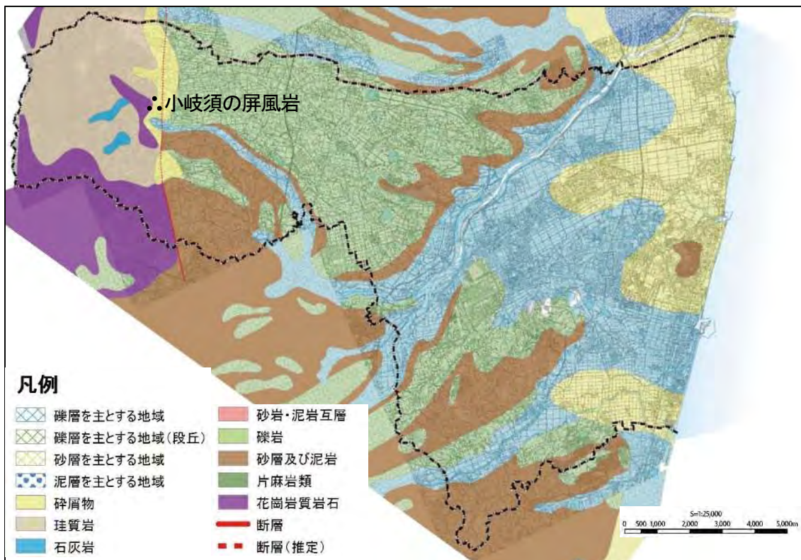
図 2-3 地質図
