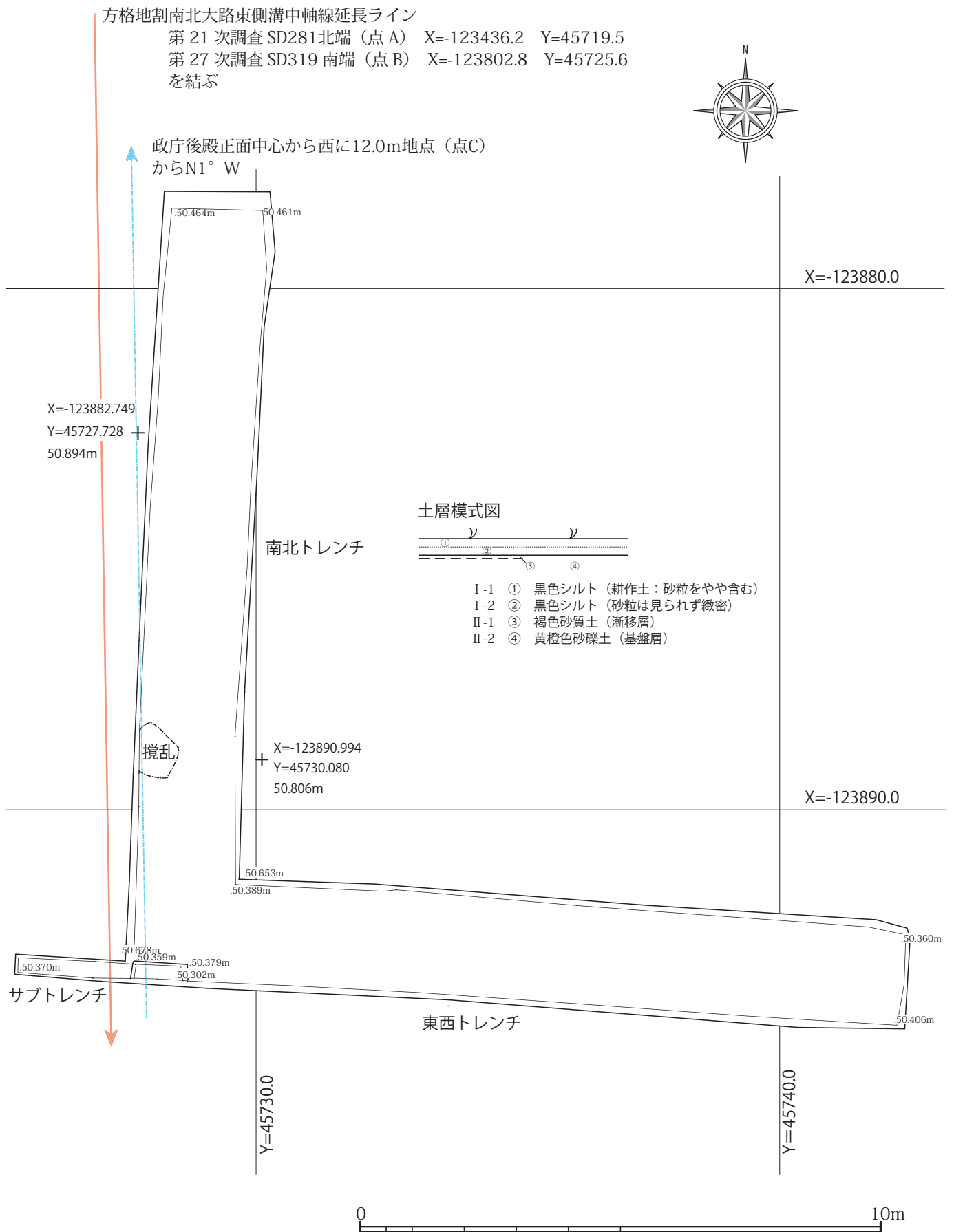
Fig.4 調査区平面図・土層模式図 1/100
