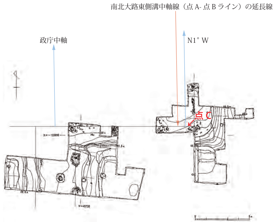
Fig.6 政庁軒廊・後殿調査区遺構配置図 1/200
