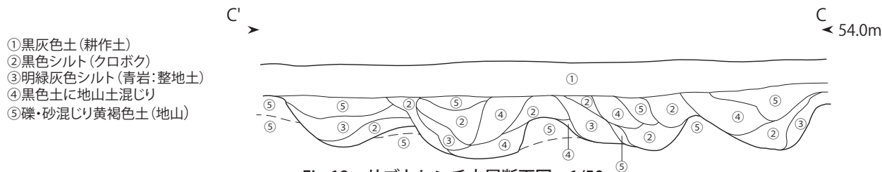
Fig.19 サブトレンチ土層断面図 1/50
