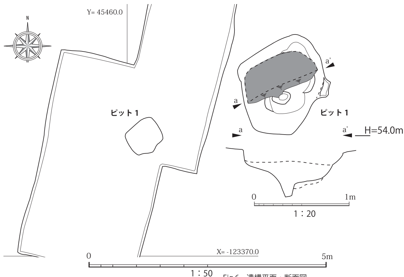
Fig.6 遺構平面・断面図
