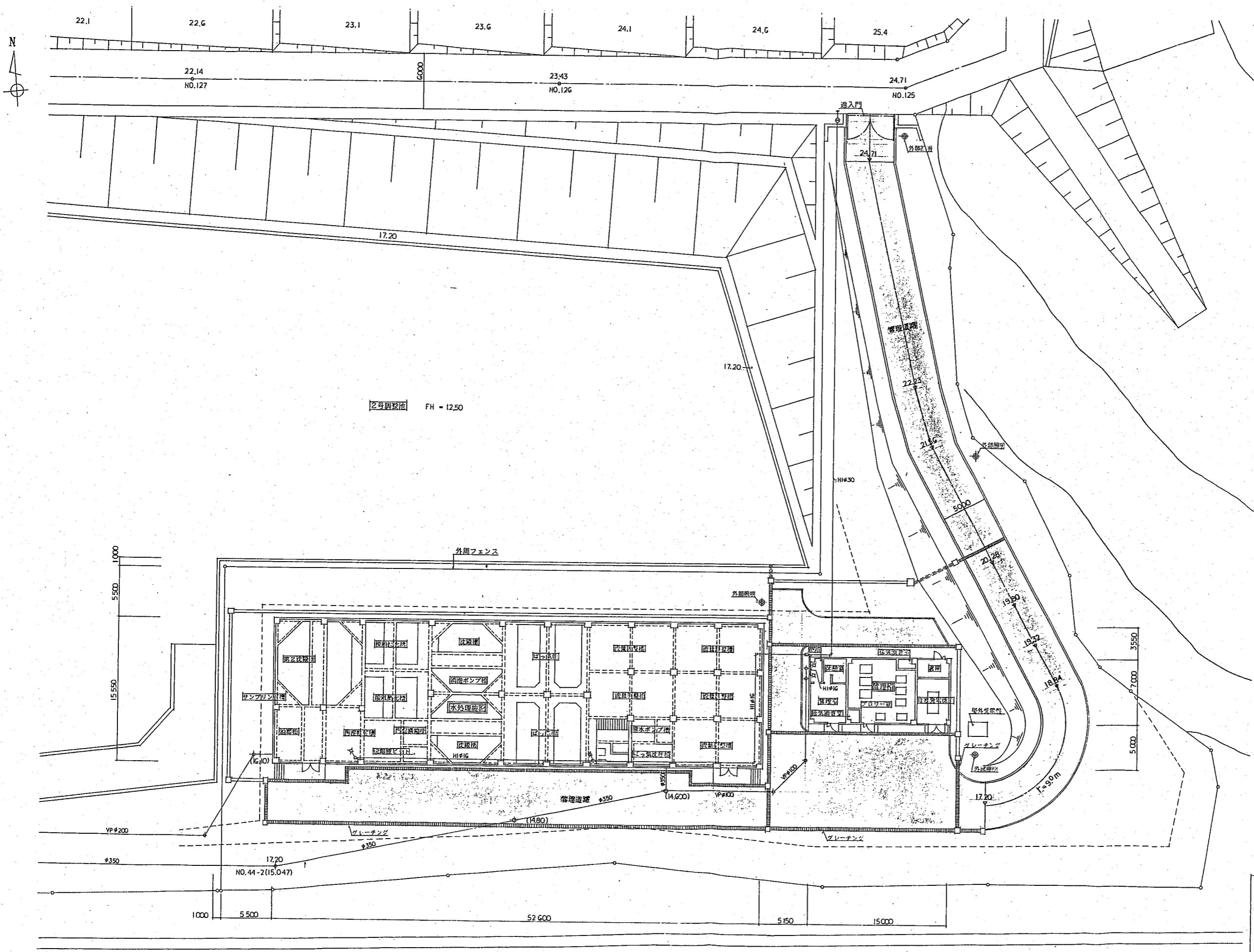
配置図 s:1/200
