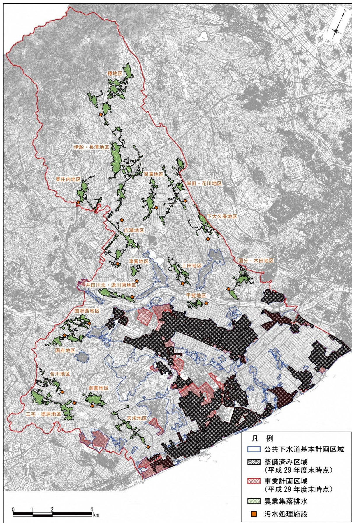
図 4-6 生活排水処理区域図
