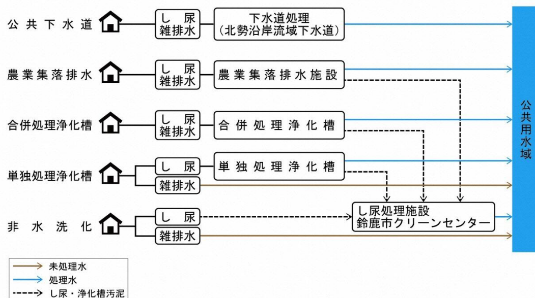
図 4-1 生活排水処理の概要
