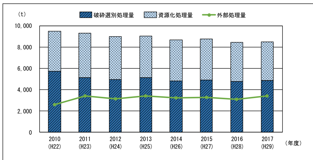
図 3-9 不燃物処理施設の処理量実績
