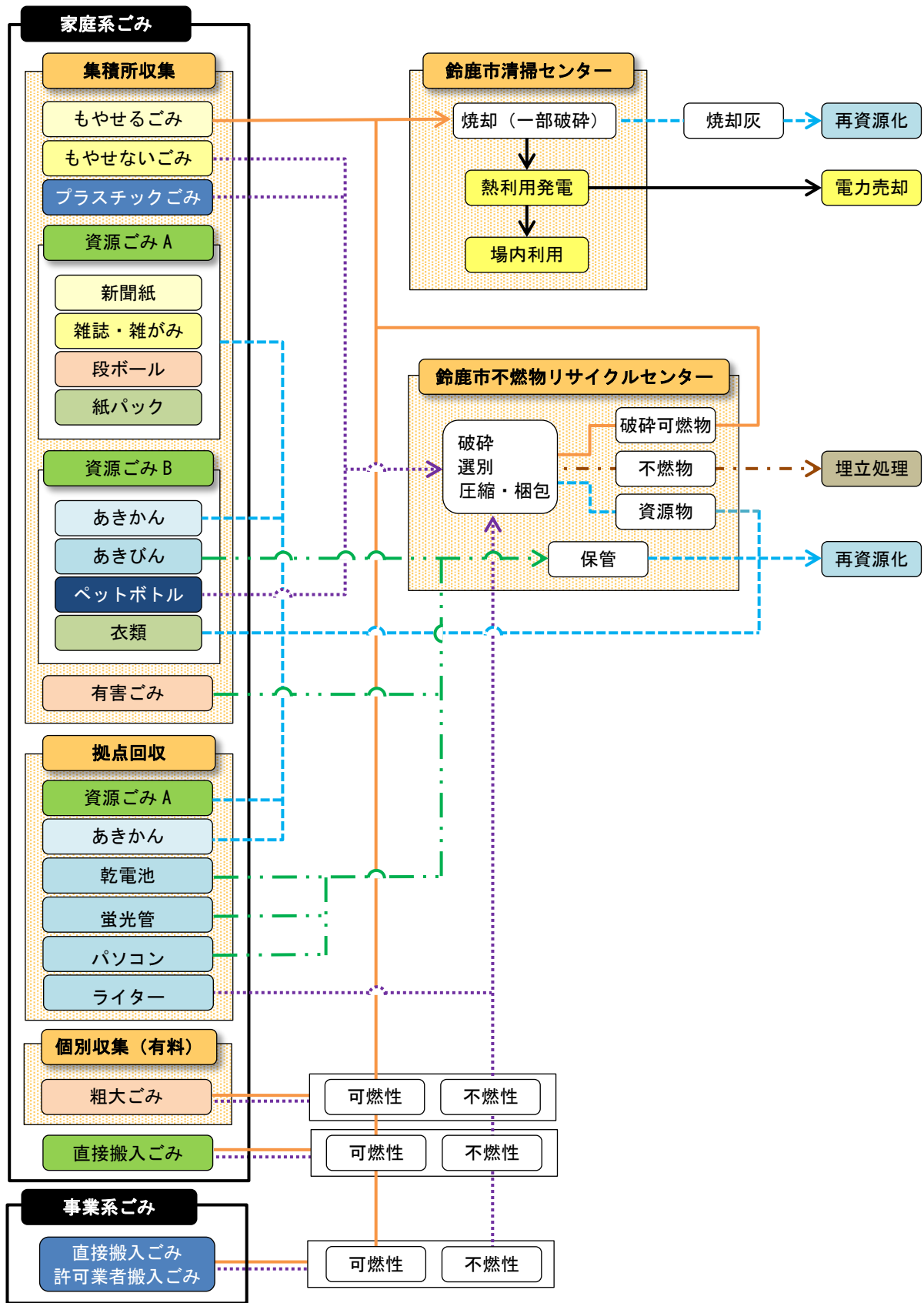
図 3-1 ごみ処理フロー
