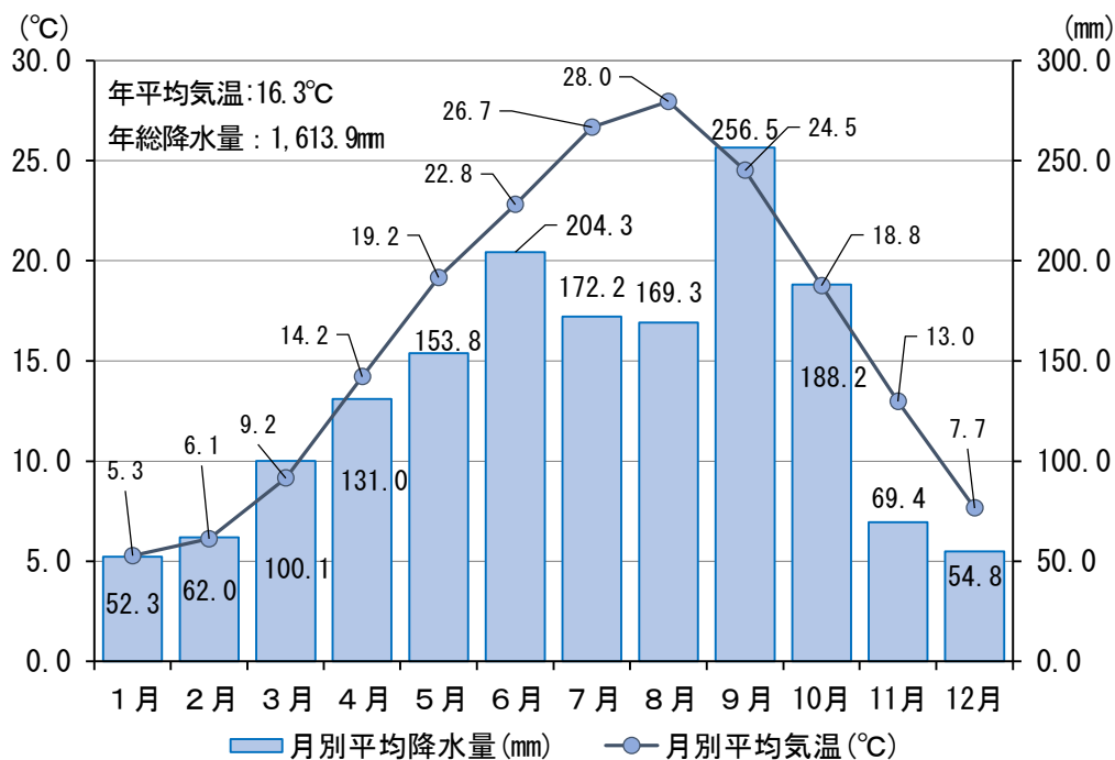
図2-5 月別平均気温・平均降水量
