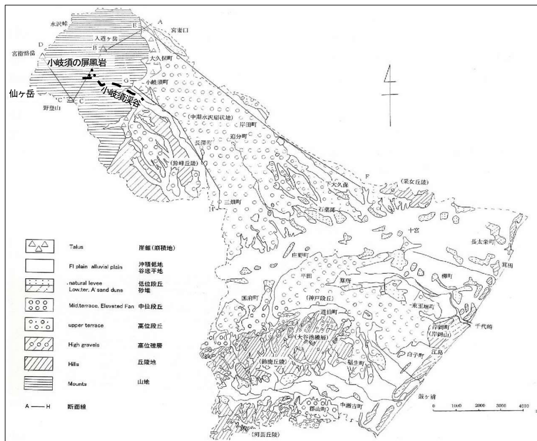
図2-2 地形分類図
