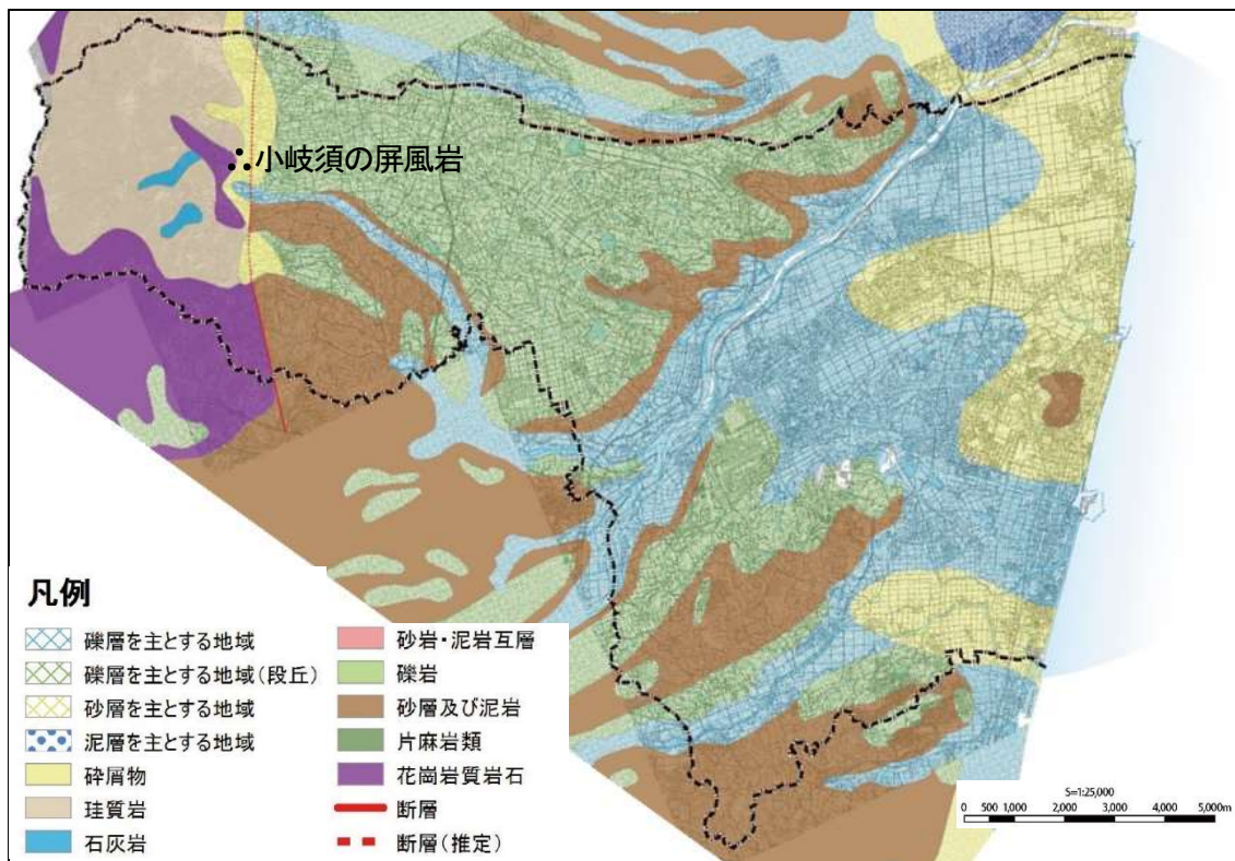
図2-3 地質図
