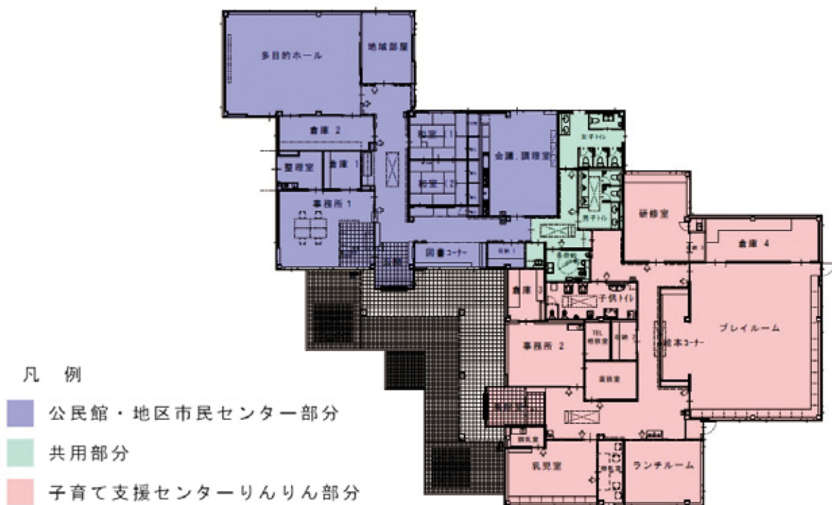
天名複合施設の平面図
