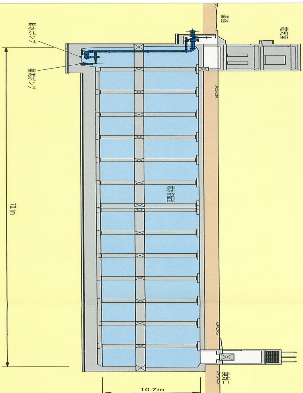
■ 新生公園雨水貯留池 断面図
