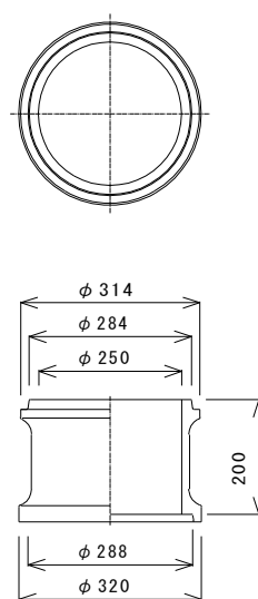
円形中部壁 H=200mm
