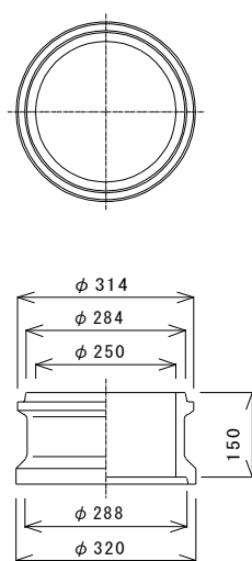
円形中部壁 H=150mm
