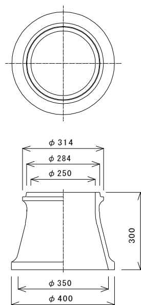
円形下部壁 H=300mm
