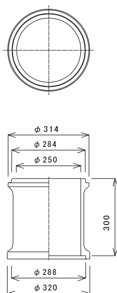
円形中部壁 H=300mm
