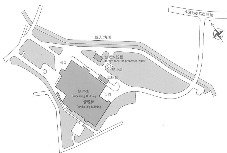
（施設配置図）
