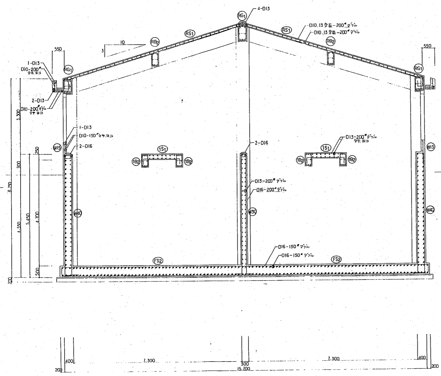
D-D 配筋詳細図 S=1/50
