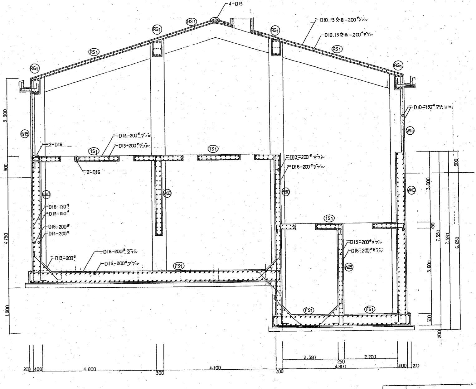
E-E 配筋詳細図 S=1/50
